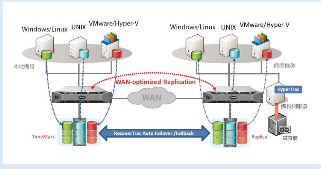
FalconStor CDP 異地備援架構圖
